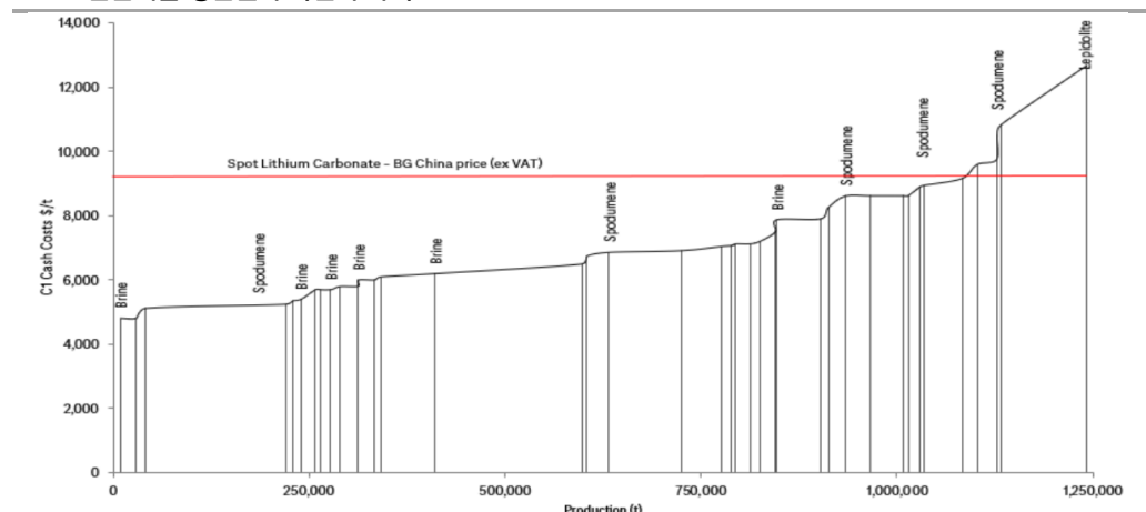
그림1 탄산리튬 생산원가 곡선과 가격
