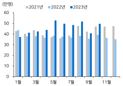
번호이동시장(MNP) 현황
