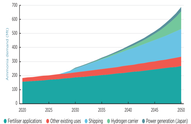
[조선] 용도별 글로벌 암모니아 수요 전망
