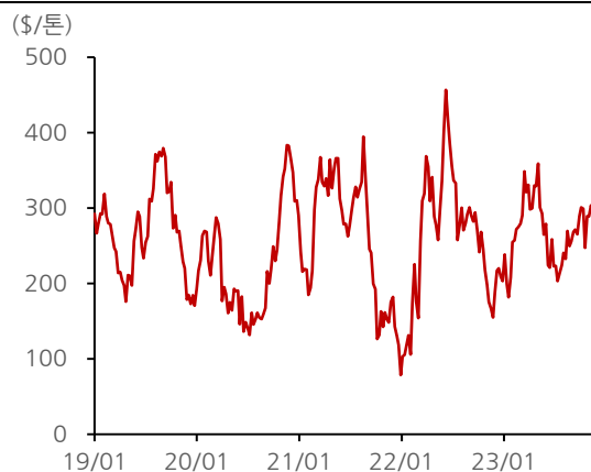
[화학] NCC 스프레드 추이
