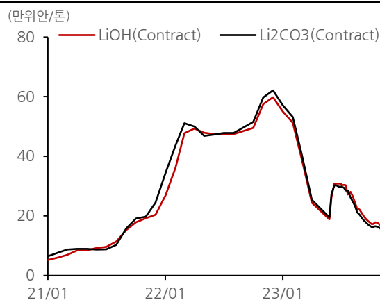
[소재] 중국 Li 2 CO 3 / LiOH 가격 추이
