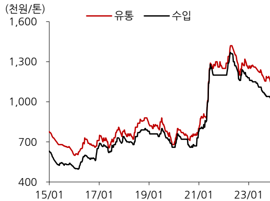
[철강] 국내 H형강 유통, 수입 가격
