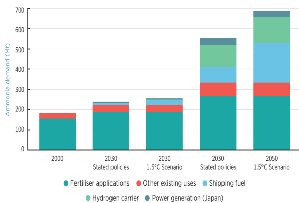
[조선] 시나리오별 글로벌 암모니아 수요 전망
