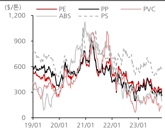
[화학] 주요 Polymer 스프레드 추이
