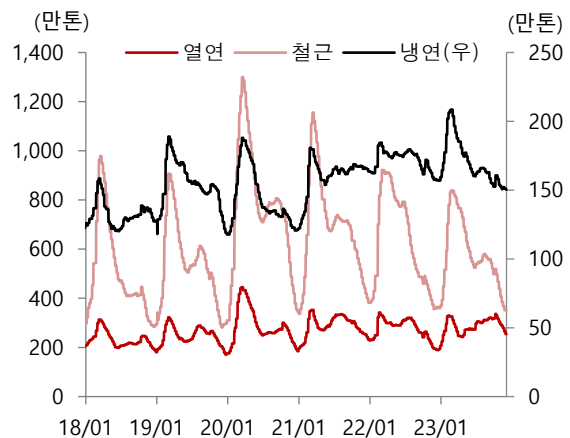
[철강] 중국 열연, 냉연, 철근 재고 추이
