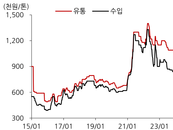
[철강] 국내 후판 유통 수입 가격
