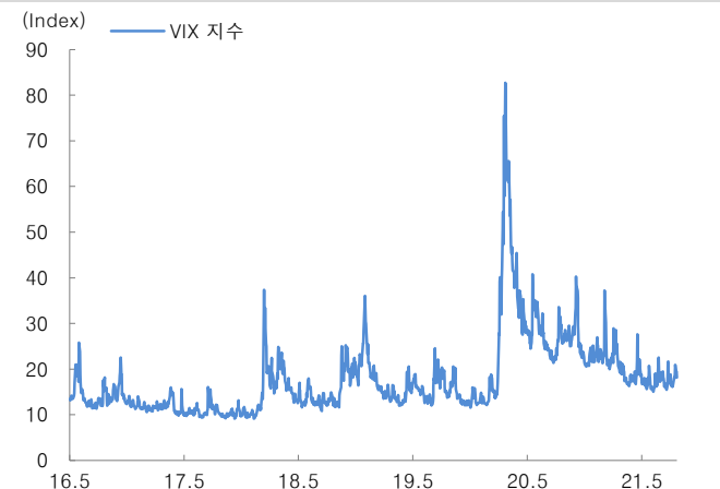
그림 12. VIX 추이
