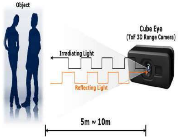
<그림8> 3D 센서 카메라 모듈(큐브아이) 기술
