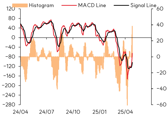
S&P 500 MACD
