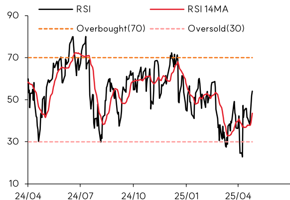
나스닥 RSI
