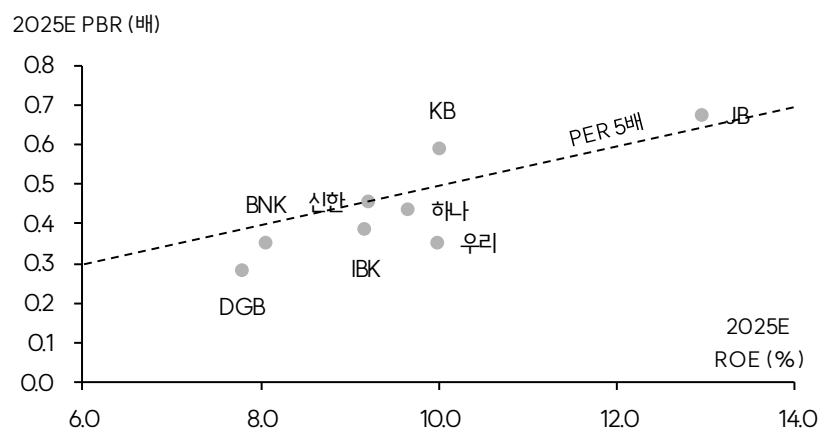
PBR-ROE Matrix (25E)
