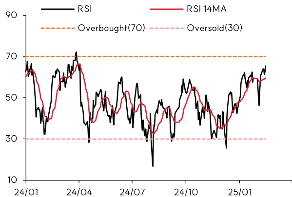
코스닥 RSI
