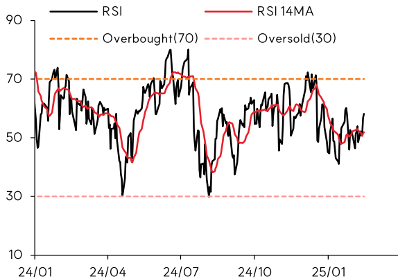
나스닥 RSI
