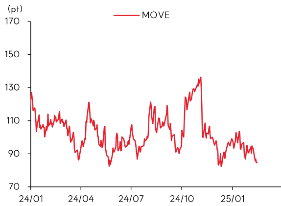
MOVE 추이
