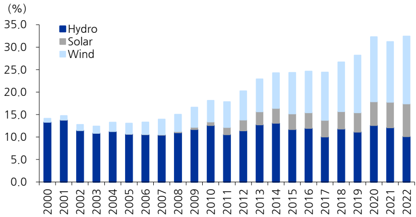
도표 1. EU의 연간 발전량 기준 재생에너지 비중 추이
