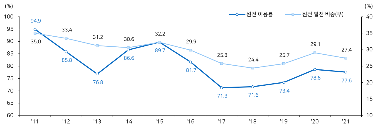
그림1 국내 원전 이용률 및 발전 비중 추이
