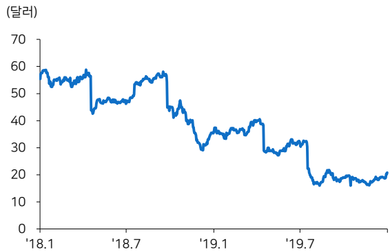
그림46 Fluor
