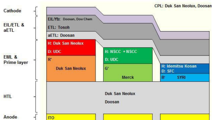
그림 5. OLED 패널 재료 구조도
