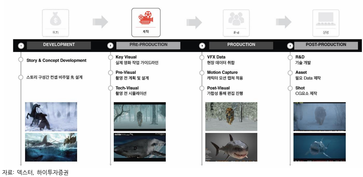
그림57. VFX Workflow
