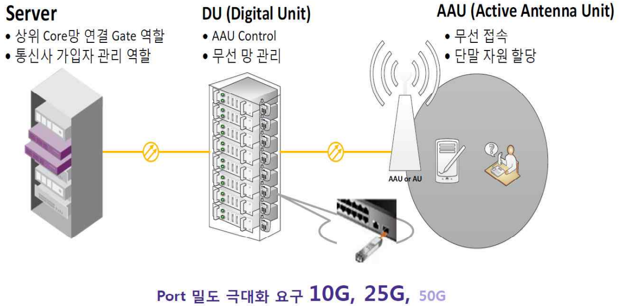
<그림 40> 5G(NR) Network Architecture (basic)
