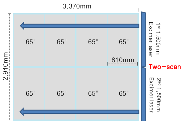
[그림 4] 10.5세대에도 LTPS (ELA 장비) 적용 가능
