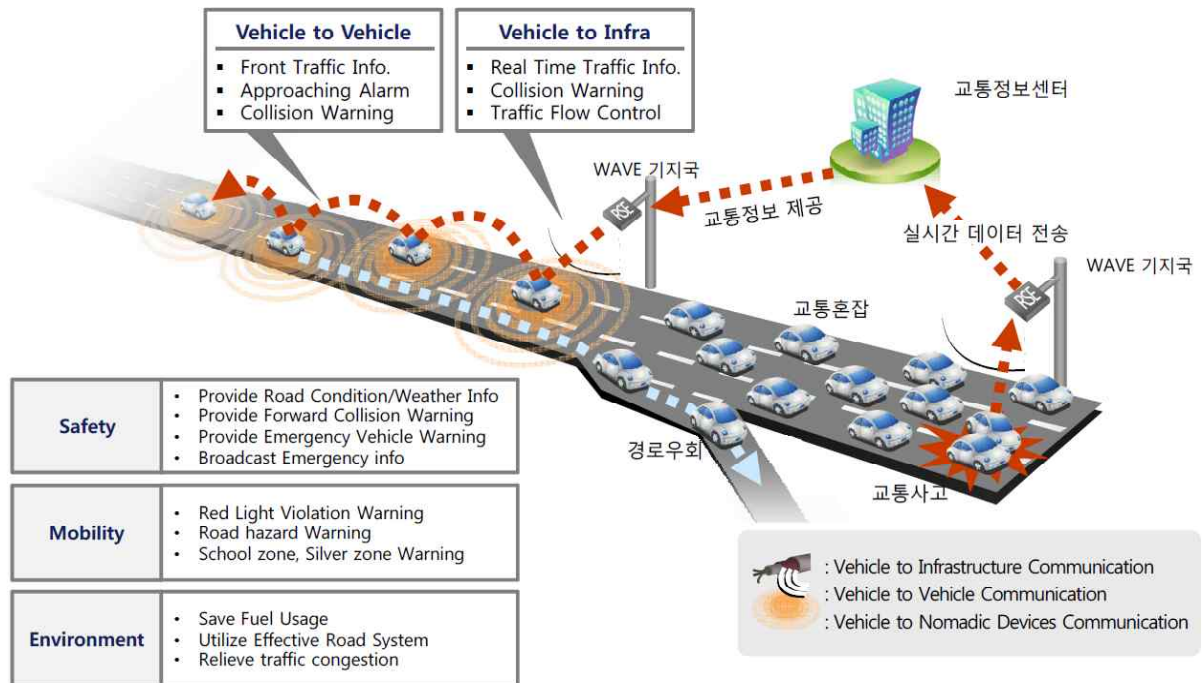
<그림 78> V2X(Vehicle-to-everything)
