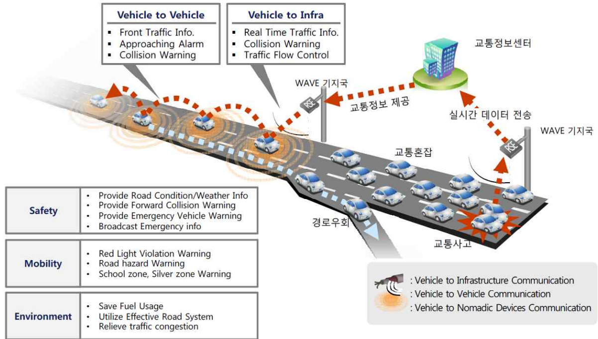
<그림 40> V2X(Vehicle-to-everything)
