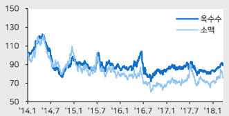
옥수수, 소맥 (2012.1.1=100)
