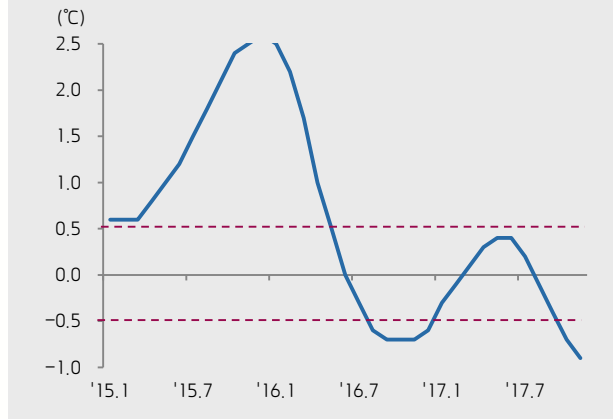
월간 ONI 지수 추이
